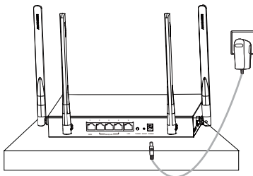
图5-2 电源连接示意图
